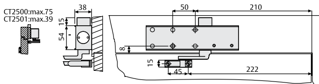
Montage inversé
