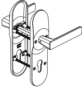
DIN LH242 Handle pair
