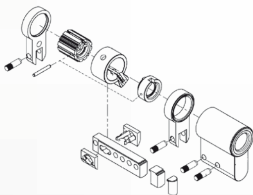
Medio Cilindro Europeo con guardapolvo eCLIQ
